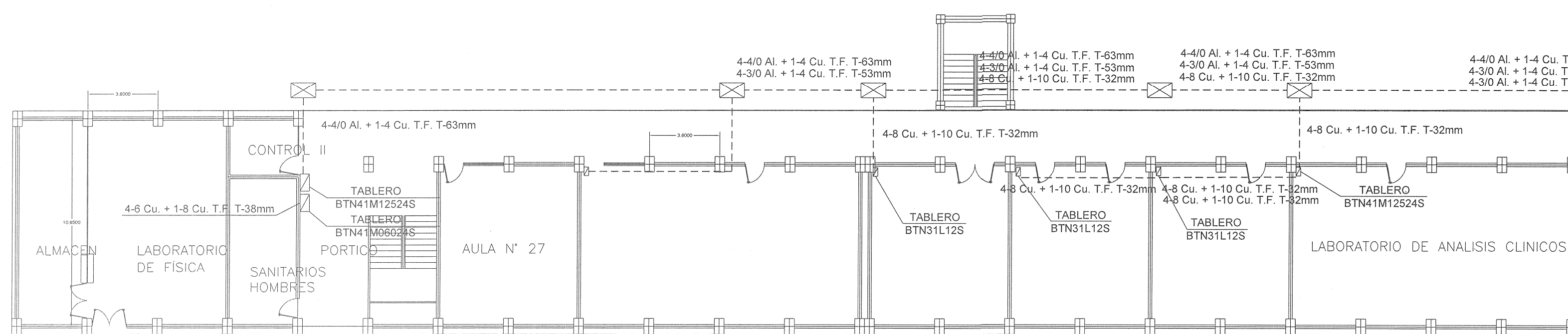
EDIFICIO "D" planta baja
