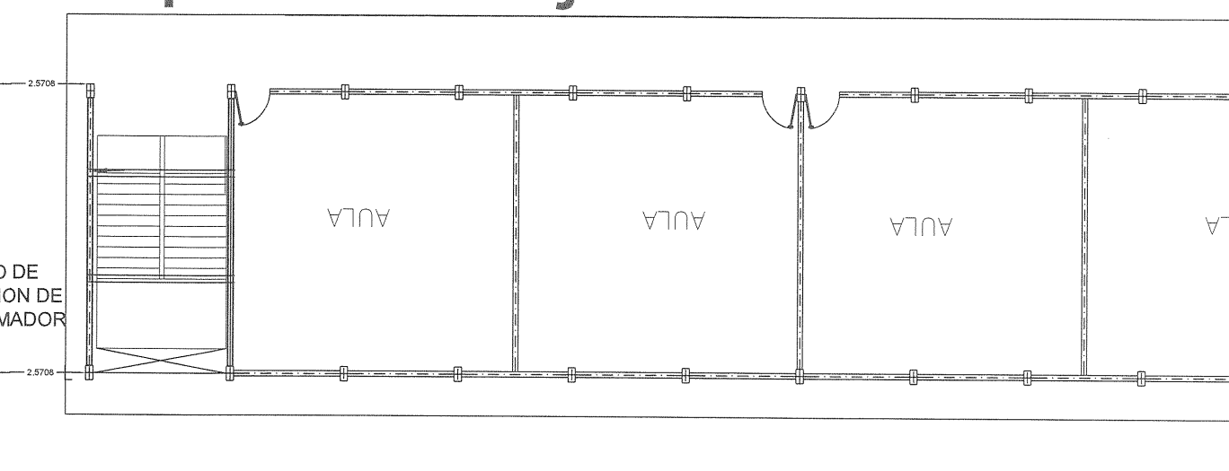
EDIFICIO "F" planta baja
