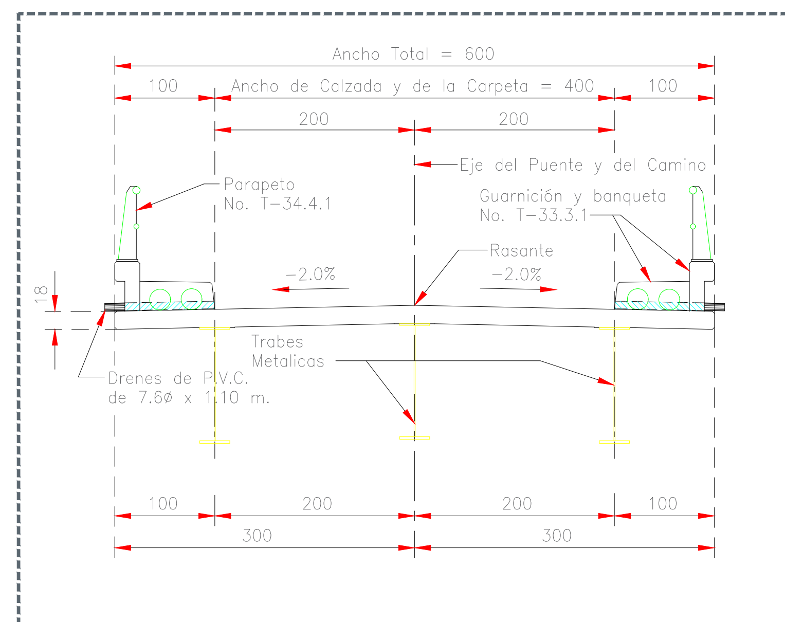
02 SECCIÓN TRANSVERSAL
