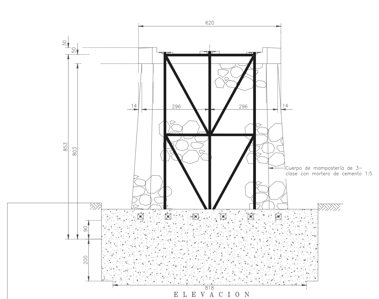
ELEVACION
